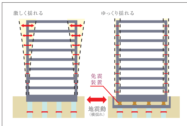
□免震構造概念図
